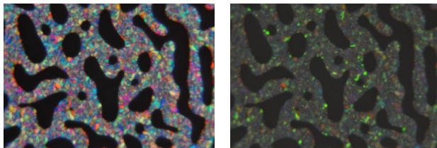
Texturen in Blue-Phase-Flüssigkristallen
